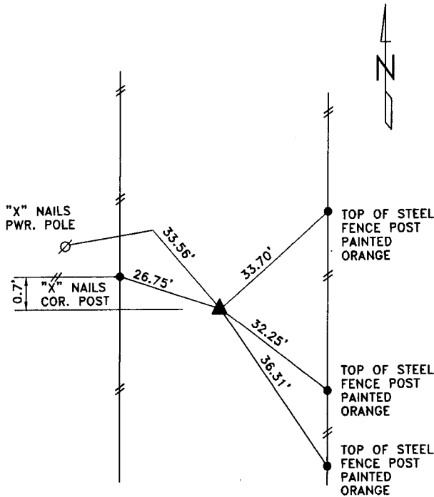
E1/4 CORNER SECTION 8-84-40
