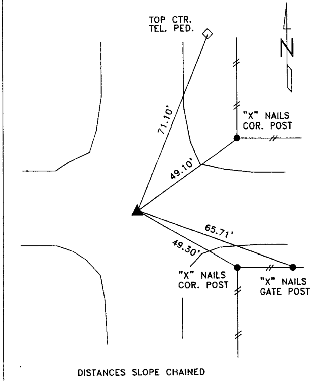
SE CORNER SECTION 26-84-40
